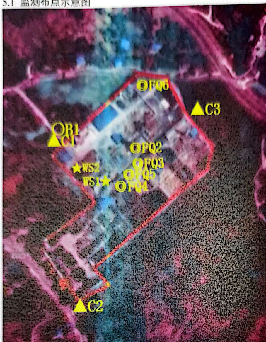
图例：★—废水（雨水）监测点，◎—有组织废气监测点，○—无组织废气监测点，▲—厂界噪声监测点
